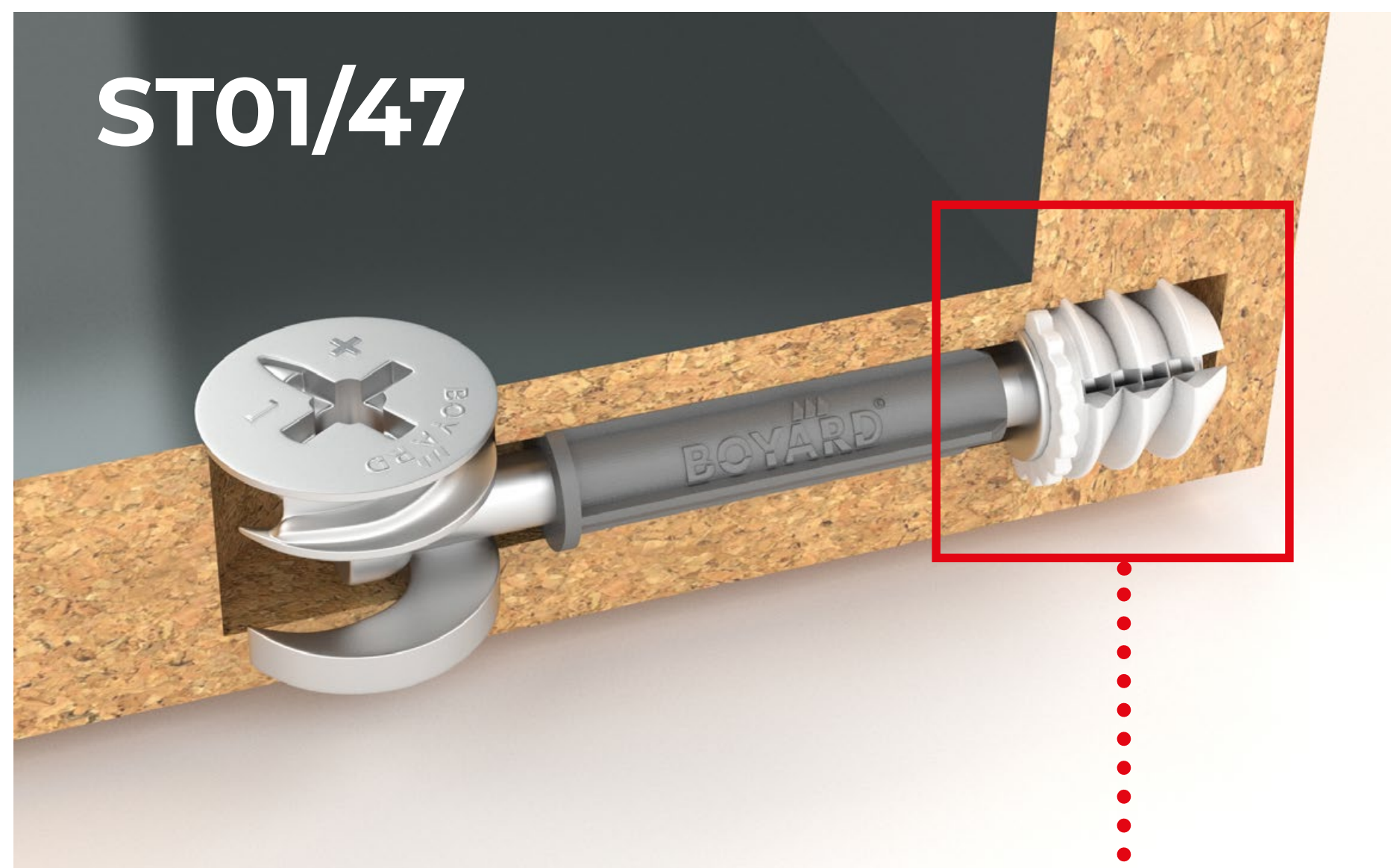
Надёжная футорка в комплекте
