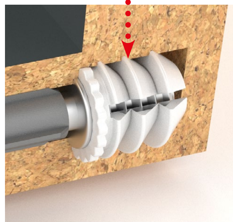
Надёжная футорка в комплекте
